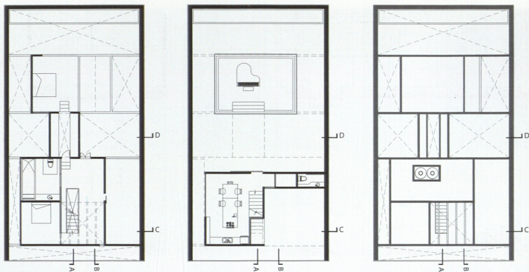
PLANTA PRIMERA, PLANTA BAJA, PLANTA DE CUBIERTAS Y SECCIONES FIRST FLOOR, GROUND FLOOR, ROOF PLAN AND SECTIONS.
